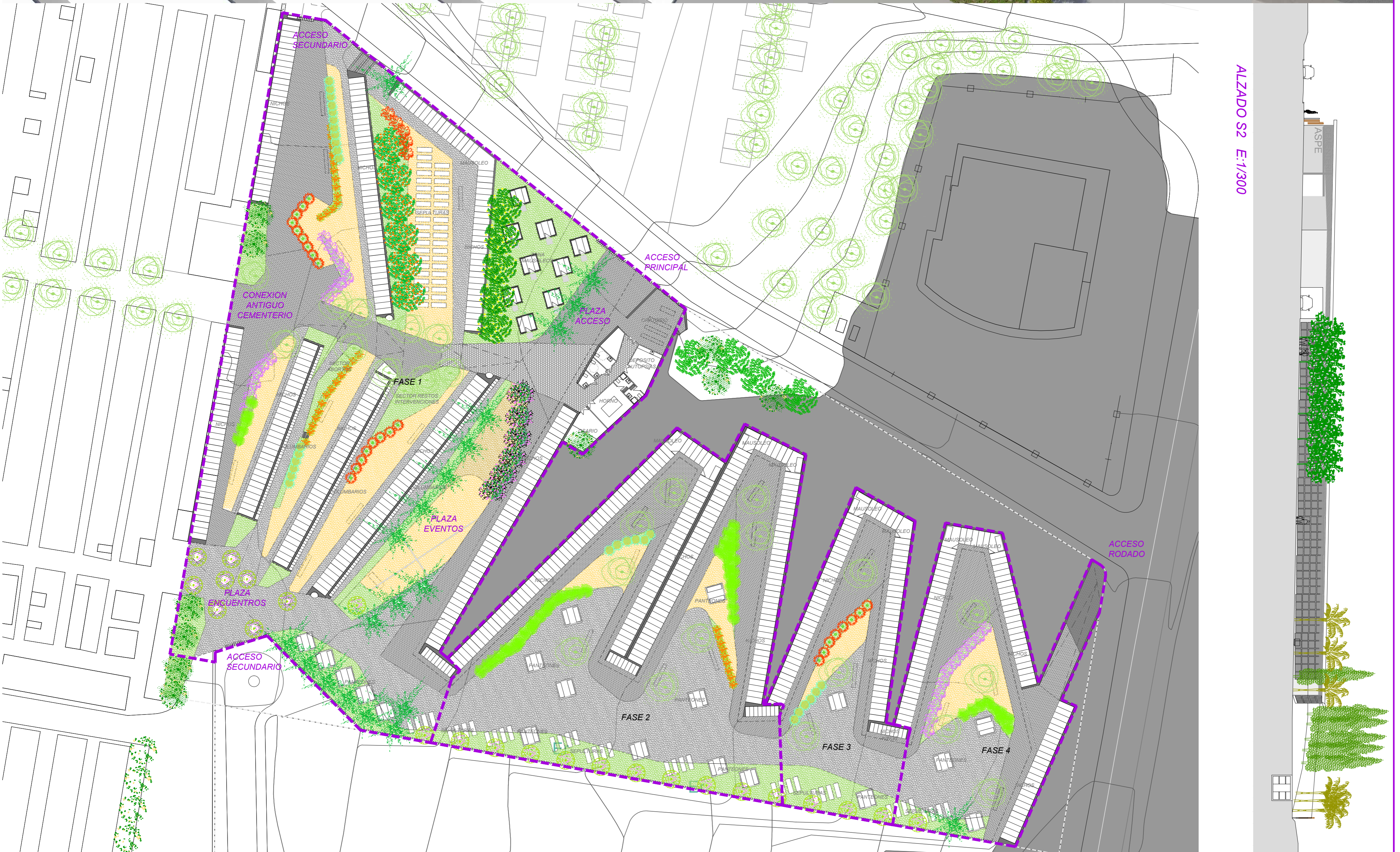
PLANTA DE ORDENACION GENERAL E:1/300
